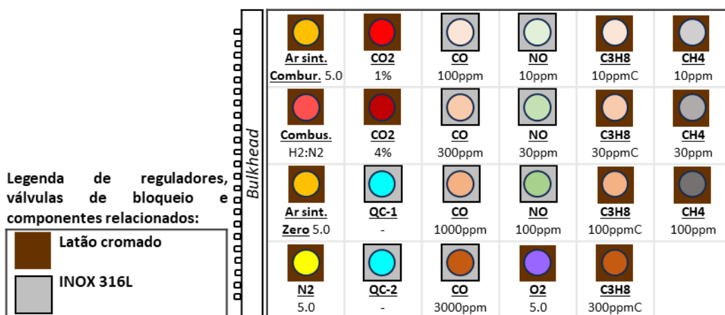
Figura 1. Representação de Painel 4 x 6, linhas x colunas, contendo 23 (vinte e três) reguladores de posto de simples estágio com válvulas de bloqueio, totalizando 14 (quatorze) reguladores e válvula de bloqueio de Latão cromado ou niquelado e 09 (nove) reguladores e válvulas de bloqueio de INOX 316L ( bulkhead optativo).
