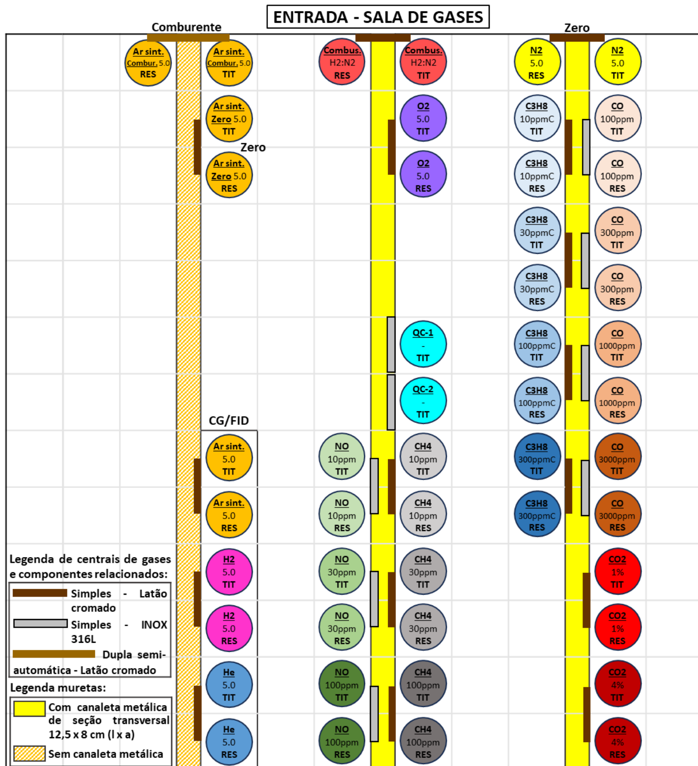
Figura 2. Representação de cilindros de gases e misturas gasosas, em pares, um principal chamado de TIT (Titular) e outro RES (Reserva), em frente a suas respectivas centrais de gases simples estágio, totalizando 16 (dezesseis) centrais de gases fonte única de Latão cromado ou niquelado, 09 (nove) centrais de gases fonte única de INOX 316L e 01 (uma) central de gás fonte dupla semiautomática com chaveamento manual de Latão cromado ou niquelado.
